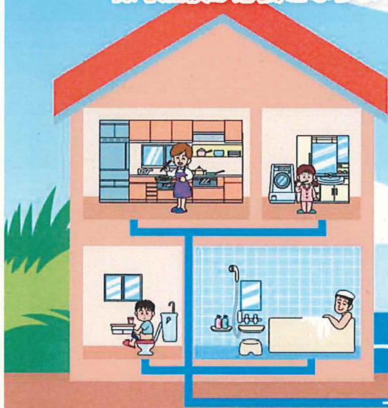
合併浄化槽 (分離接触ばっ気方式)
